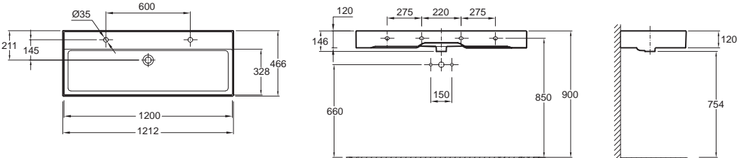
Cotas no válidas para instalación con mueble / Dimensões não válidas para a instalação com mobiliário.
